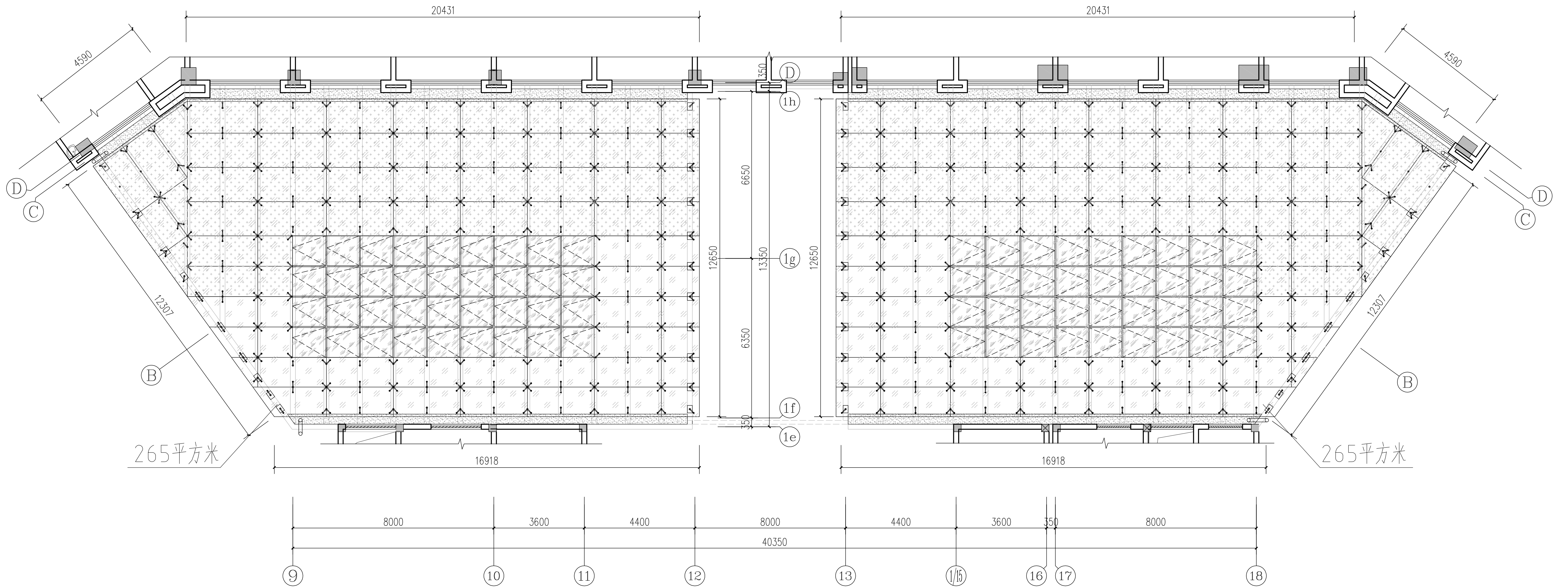
钢结构玻璃采光顶平面分格图 1:100
